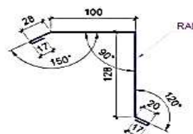
Планка ендовая декор. ТИП 2
