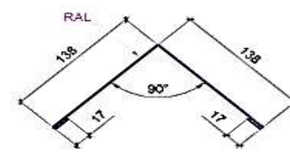
Планка карнизная ТИП 3
