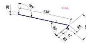
Планка ветровая для защиты карниза
