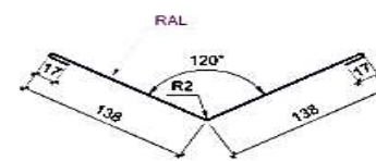
Планка ендовая декор. ТИП 3
