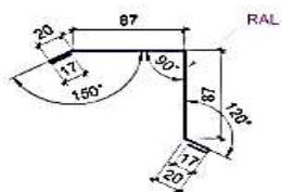
Планка ветровая ТИП 6
