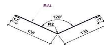
Планка ендовая декор. ТИП 3
