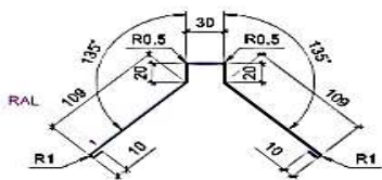
Планка конька ТИП 7
