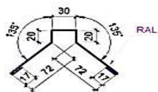
Планка карнизная ТИП 4
