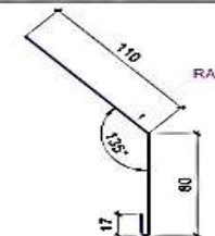
Планка ветровая ТИП 4
