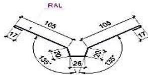
Планка ендовая декор. ТИП 1
