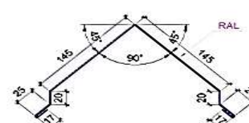
Планка карнизная ТИП 2
