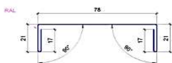
Планка выравнивающая ТИП 2
