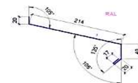
Торцевая планка для битумной черепицы
