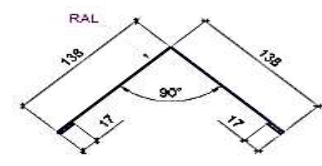
Планка карнизная ТИП 3
