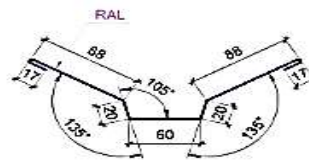
Планка ендовая декор. ТИП 2
