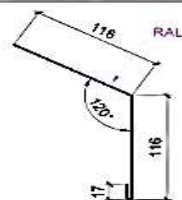
Планка ветровая ТИП 6
