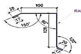
Планка ендовая декор. ТИП 2
