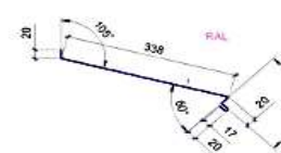
Планка ветровая для защиты карниза
