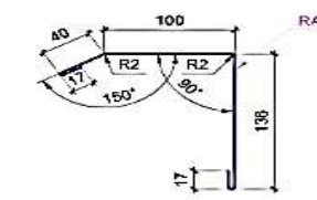
Планка ендовая декор. ТИП 4
