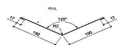
Планка ендовая декор. ТИП 4
