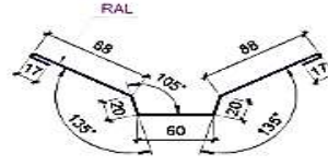
Планка ендовая декор. ТИП 2
