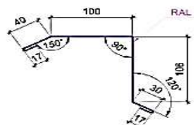
Планка ендовая декор. ТИП 1
