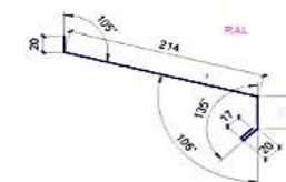
Торцевая планка для битумной черепицы
