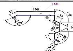
Планка ендовая декор. ТИП 3
