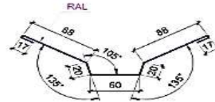
Планка ендовая декор. ТИП 2
