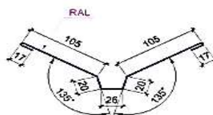
Планка ендовая декор. ТИП 1
