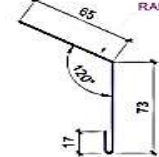
Планка ветровая ТИП 3
