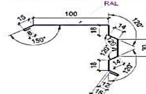
Планка ендовая декор. ТИП 3
