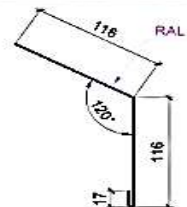
Планка ветровая ТИП 6
