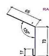
Планка ветровая ТИП 3
