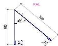
Планка для битумной черепицы
