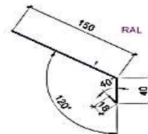
Планка ветровая ТИП 2
