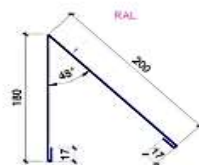
Планка для битумной черепицы
