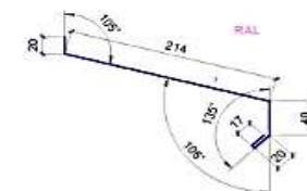
Торцевая планка для битумной черепицы
