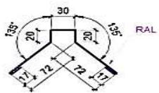
Планка карнизная ТИП 4
