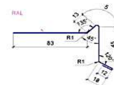
Торцевая планка для битумной черепицы
