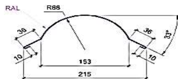
Планка ветровая ТИП 1
