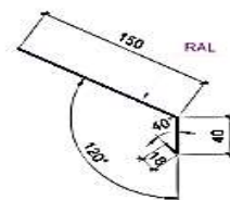
Планка ветровая ТИП 2
