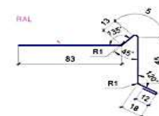
Торцевая планка для битумной черепицы
