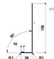
Планка ветровая для защиты карниза
