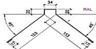
Планка карнизная ТИП 1
