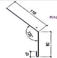
Планка ветровая ТИП 4
