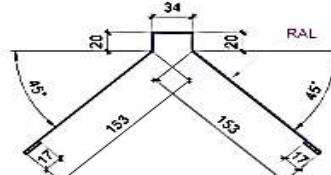
Планка карнизная ТИП 1
