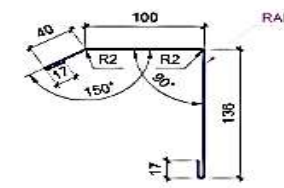
Планка ендовая декор. ТИП 4
