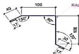
Планка ендовая декор. ТИП 1
