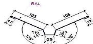
Планка ендовая декор. ТИП 1
