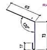
Планка ветровая ТИП 3
