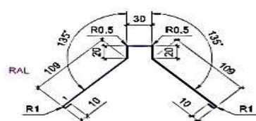
Планка конька ТИП 7
