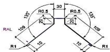
Планка конька ТИП 7
