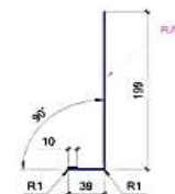
Планка ветровая для защиты карниза
