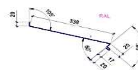
Планка ветровая для защиты карниза
