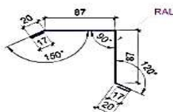
Планка ветровая ТИП 6
