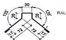
Планка карнизная ТИП 4
