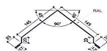
Планка карнизная ТИП 2
