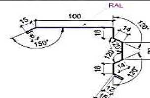
Планка ендовая декор. ТИП 3
