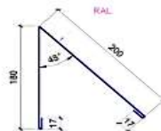
Планка для битумной черепицы
