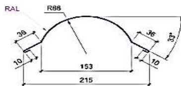
Планка ветровая ТИП 1
