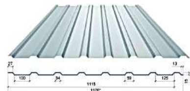
C-15 сторона Б
