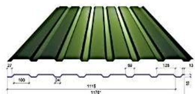
C-15 сторона А
