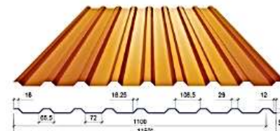
C-18 сторона Б
