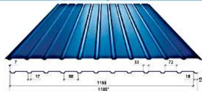
C-12 сторона А
