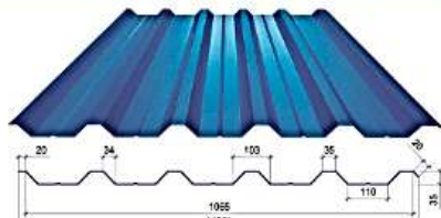
H-35 сторона А
