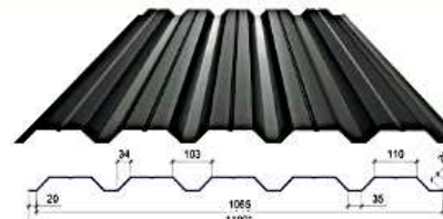
H-35 сторона Б
