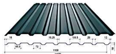
C-18 сторона А
