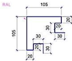
Н-планка
