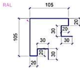
Н-планка
