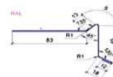
Торцевая планка для битумной черепицы
