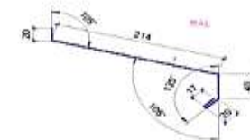
Торцевая планка для битумной черепицы
