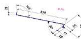
Планка ветровая для защиты карниза
